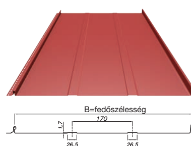
Lindab SRP Click Dn
